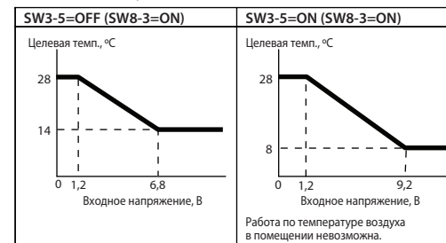
Тип зависимости Б (режим „Нагрев”)
