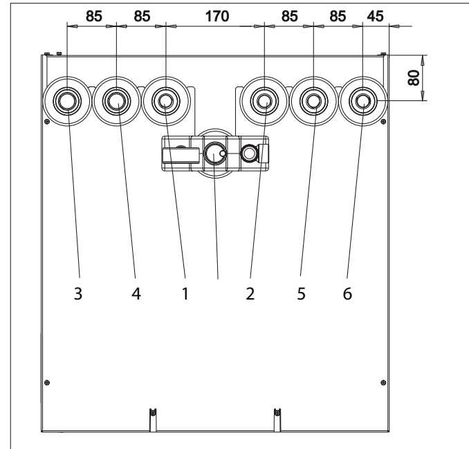
Подключение гидро модуля (вид сверху)
