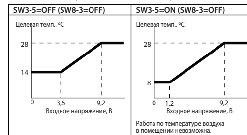
Тип зависимости Б (режим „Охлаждение”)
